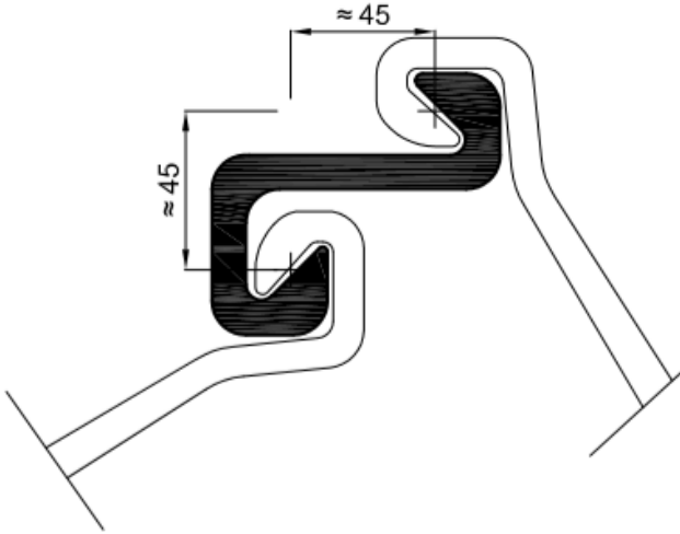
E20 15.38 kg/m
