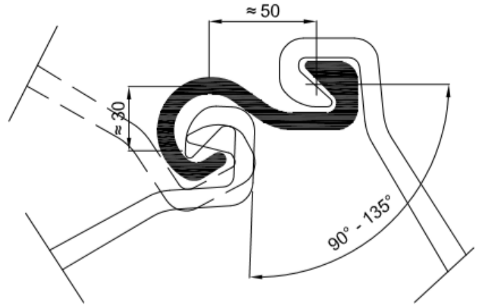
E20-XL 12.02 kg/m
