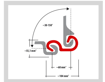
VTSn (LTn) - 15,5 kg/m
