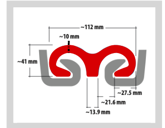
M20 (V20) - 13,63 kg/m
